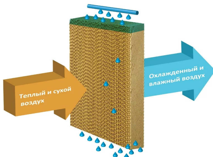
Рис. 2.83. Принцип работы ОУ ИТ (clck.ru/34NvVe)
