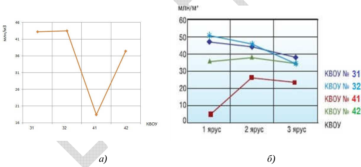
Рис. 5.27. Распределение количества частиц в кубометре атмосферного воздуха: а) перед КВОУ; б) по ярусам КВОУ
