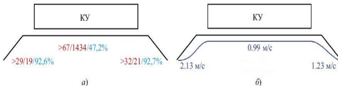
Рис. 5.4. Результаты мониторинга потока атмосферного воздуха на всасах КВОУ 13.05.2016: а) количество, концентрация и процентное содержание мелкодисперсных частиц 0,3 мкм; б) скорость потока атмосферного воздуха на всасах КВОУ
