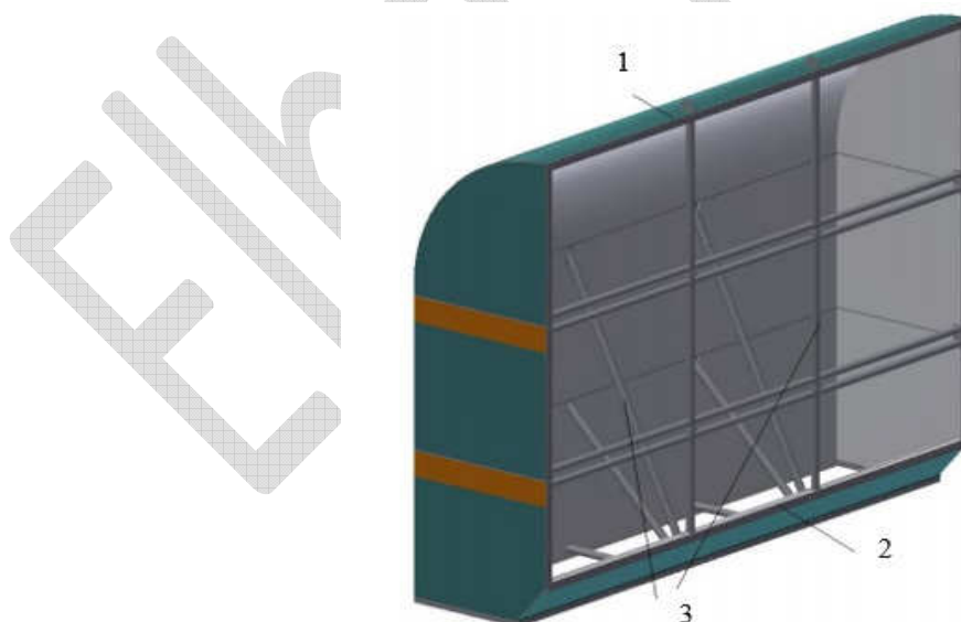
Рис. 3.32. Конструкция углового воздухопровода: 1 – угловой воздуховод; 2 – дефлектор; 3 – трубы жесткости
