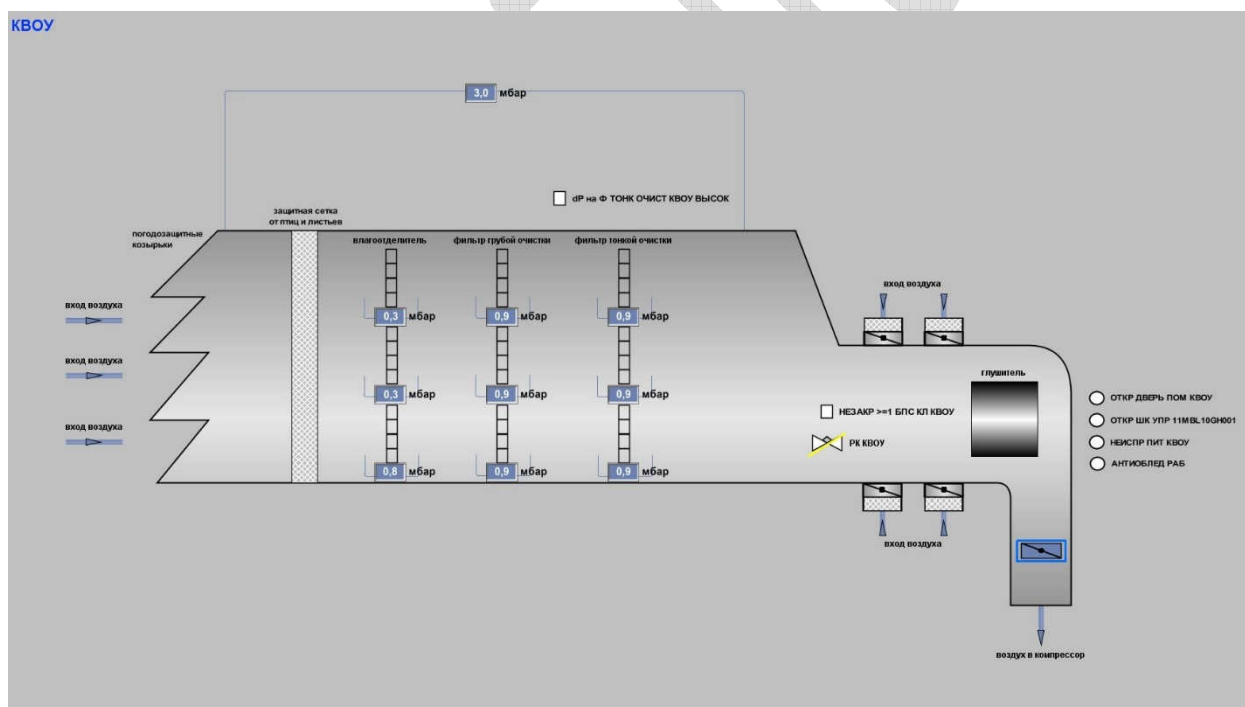
Рис.4.37. Мнемокадр показаний датчиков давления на всех ярусах КВОУ ГТЭ-160
