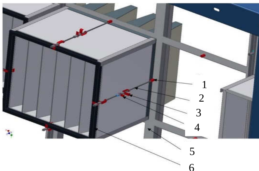
Рис. 3.27. Крепление рамки фильтрующего модуля с элементами ФГО: 1 – накатные гайки; 2 – резьбовой стержень; 3 – крепёжный угол; 4 – крепёжная пластина; 5 – короб; 6 – рамка
