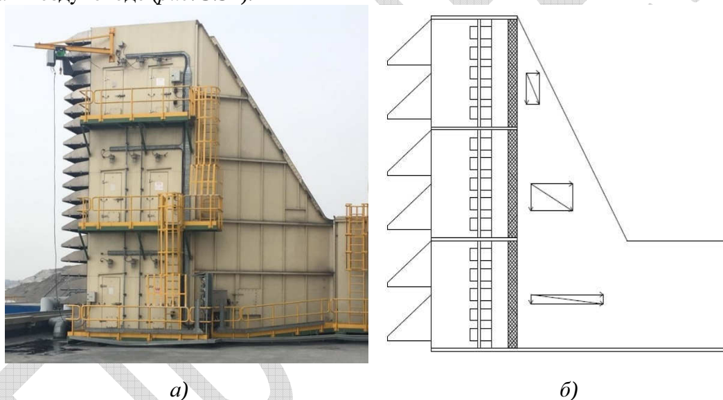
Рис. 5.34. КВОУ В: а) воздуховод на уровне верхнего яруса КВОУ; б) схема КВОУ и воздуховода с треугольниками скоростей после фильтров
