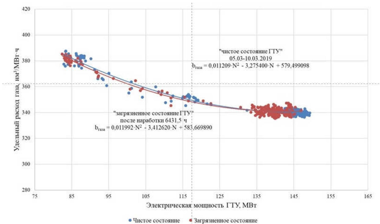
Рис. 4.34. Зависимость удельного расхода топливного газа от мощности ГТУ-32
