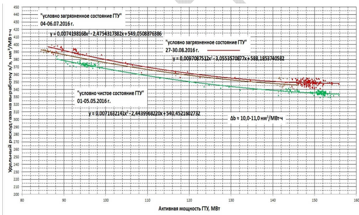
Рис. 4.29. График отклонения расходной характеристики ГТУ-31 V94.2 ТЭЦ в МО вследствие загрязнения проточной части осевого компрессора
