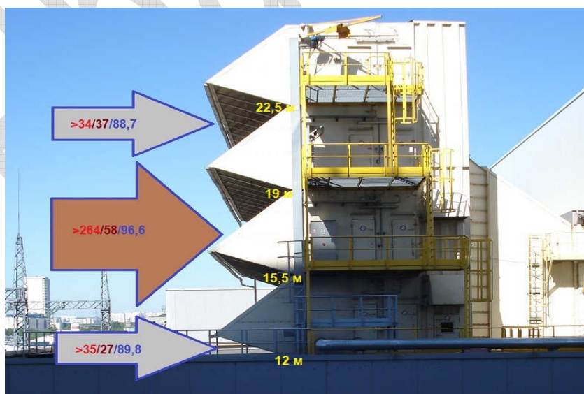
Рис. 4.7. Распределение слоев воздуха на всасе КВОУ ГТУ ТЭЦ 2 в ЮАО: первое число – суммарное количество взвешенных частиц; второе – суммарная концентрация взвешенных частиц; третье – процентное содержание мелкодисперсных частиц 0,3 мкм в кубометре воздуха
