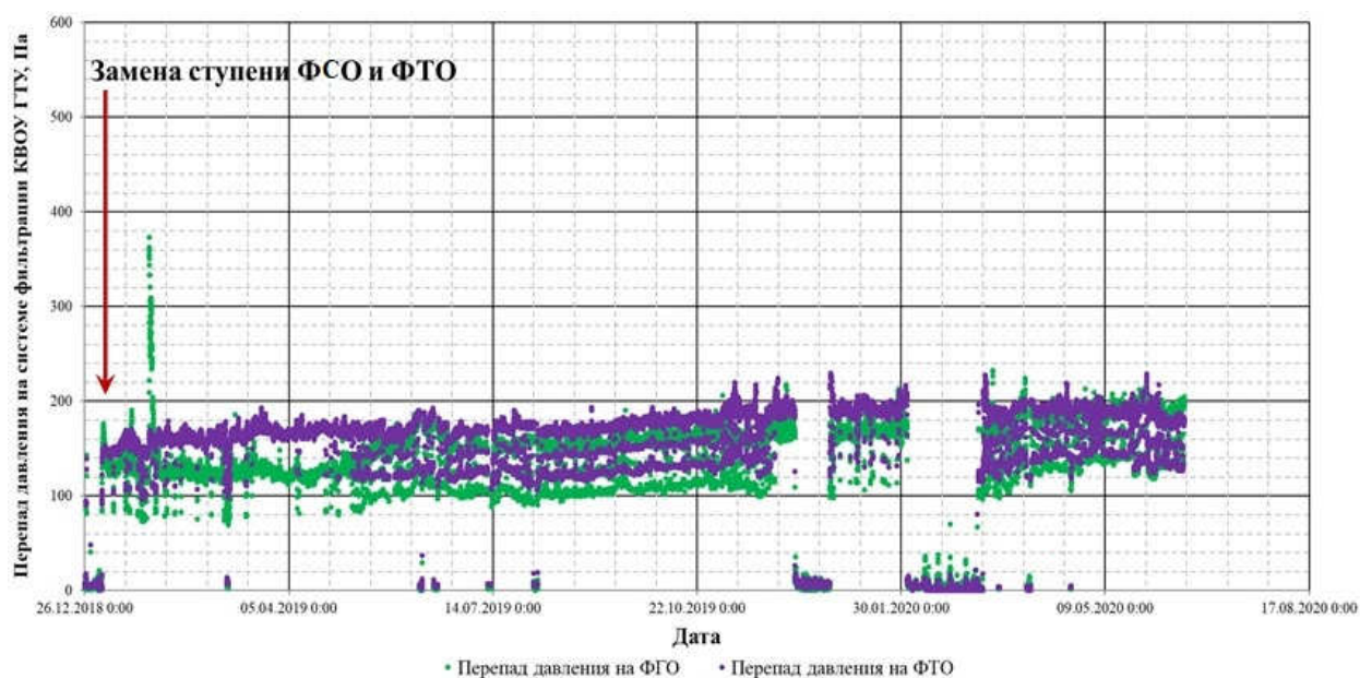
Рис. 4.32. Тренды перепадов давления на фильтрах КВОУ ГТУ-32
