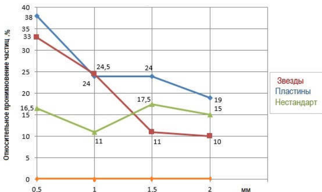
Рис. 2.22. Графики проникновения снежинок на верхний ярус КВОУ
