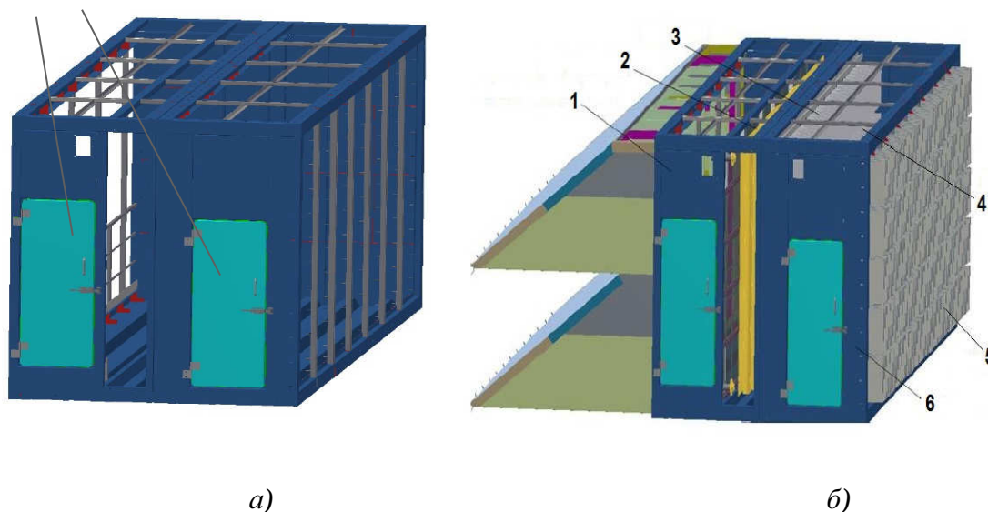
Рис. 3.24. Модули КВОУ ГТУ: а) неоснащенный; б) оснащенный: 1 – секция предподогрева воздуха (трубопроводы); 2 – секция теплообменного аппарата; 3 – секция коагуляторов; 4 – секция префильтров; 5 – секция ФТО; 6 – секция фильтров
