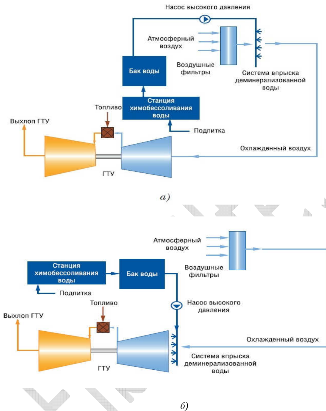
Рис. 2.86. Принципиальная схема системы охлаждения воздуха с впрыском ХОВ: а) после системы фильтрации КБОУ; б) на всасе в осевой компрессор ГТУ
