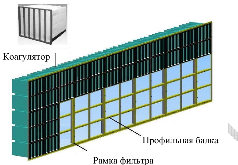
Рис. 3.26. Модуль для установки коагуляторов
