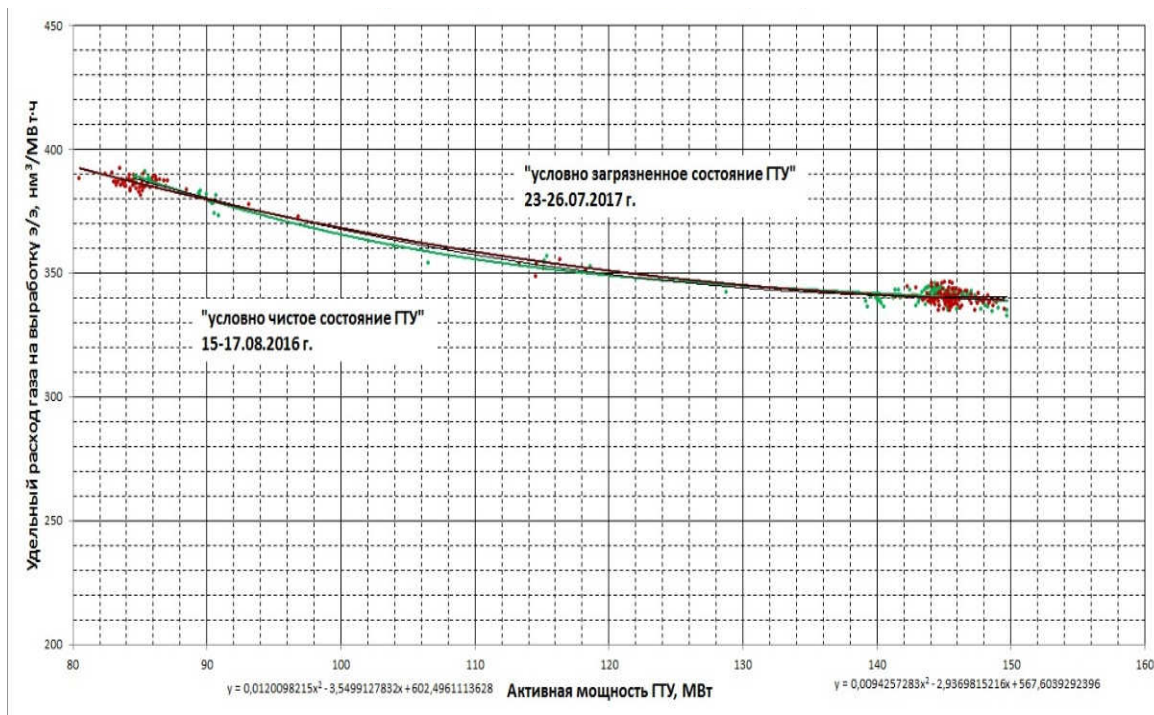
Рис. 4.26. График отклонение расходной характеристики ГТУ-32 V94.2 ТЭЦ в МО вследствие загрязнения проточной части осевого компрессора
