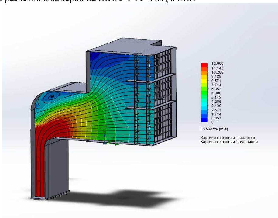
Рис. 5.22. Картина течения воздушного потока по высоте КВОУ ГТУ ТЭЦ
