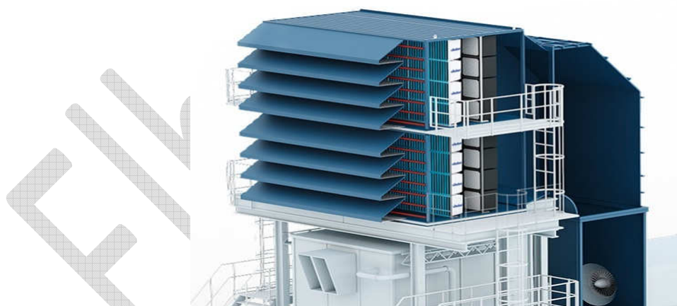
Рис. 3.12. 3D КВОУ с двухступенчатой системой фильтрации и ИК-обогревателями (рис. из буклета компании Freudenberg Filtration Technologies)
