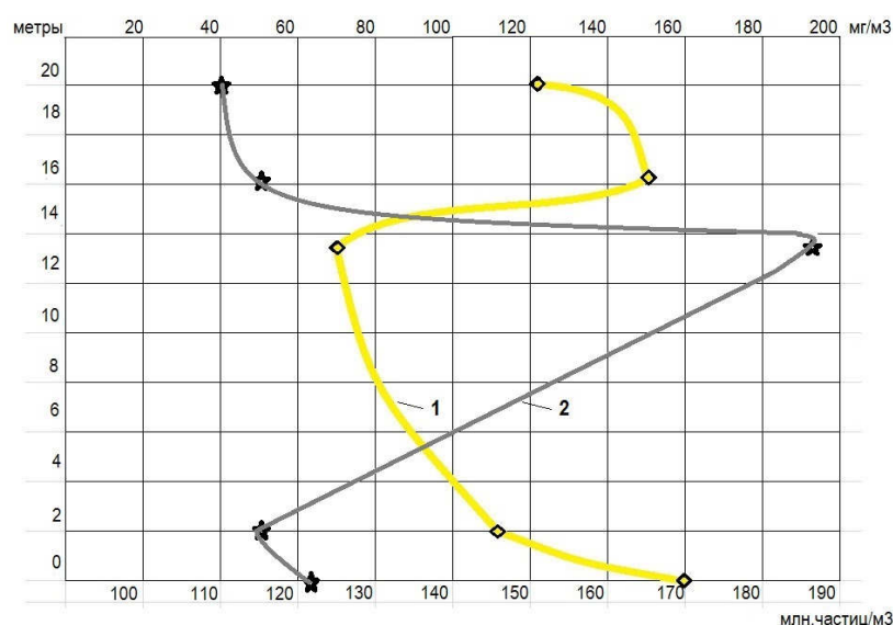
Рис. 4.4. Распределение суммарного количества (1) и концентрации (2) взвешенных частиц в кубометре атмосферного воздуха по высоте КВОУ (19.11.2015)
