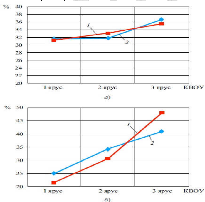
Рис. 5.10. Распределение концентрации (1) и количества (2) частиц в кубометре атмосферного воздуха по ярусам: а) КВОУ Б; б) КВОУ В ТЭЦ в САО
