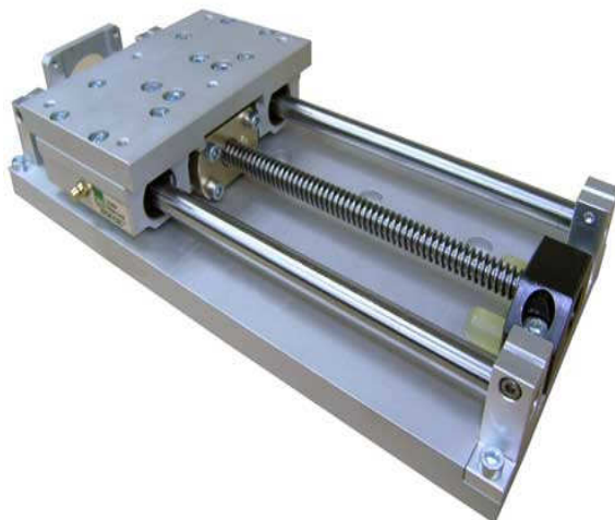
Рис. 2.61. Модуль линейного перемещения (фото из буклета Завода мехатронных изделий)
