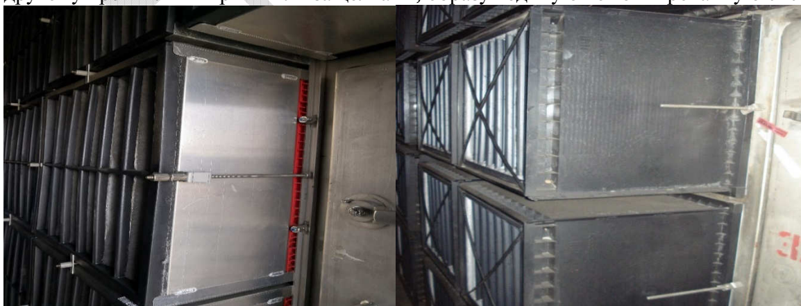
Рис. 3.15. Короба комбисистем: а) компании FAIST AIS из нержавеющей стали; б) компании Mikrogor из пластмассы
