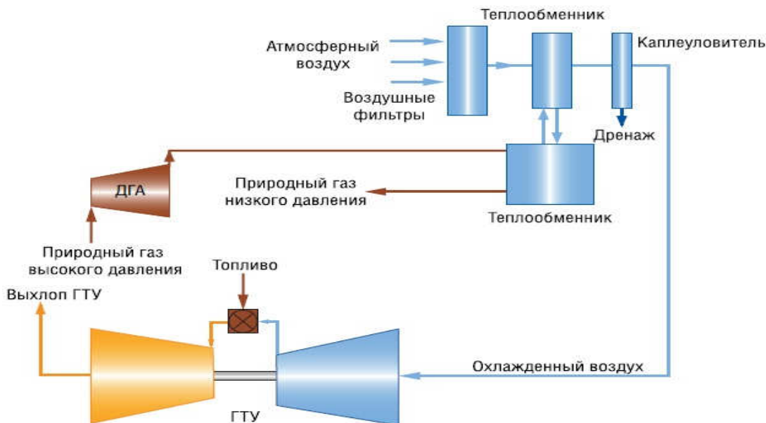
Рис. 2.89. Принципиальная схема системы охлаждения циклового воздуха с помощью турбодетандеров [21]
