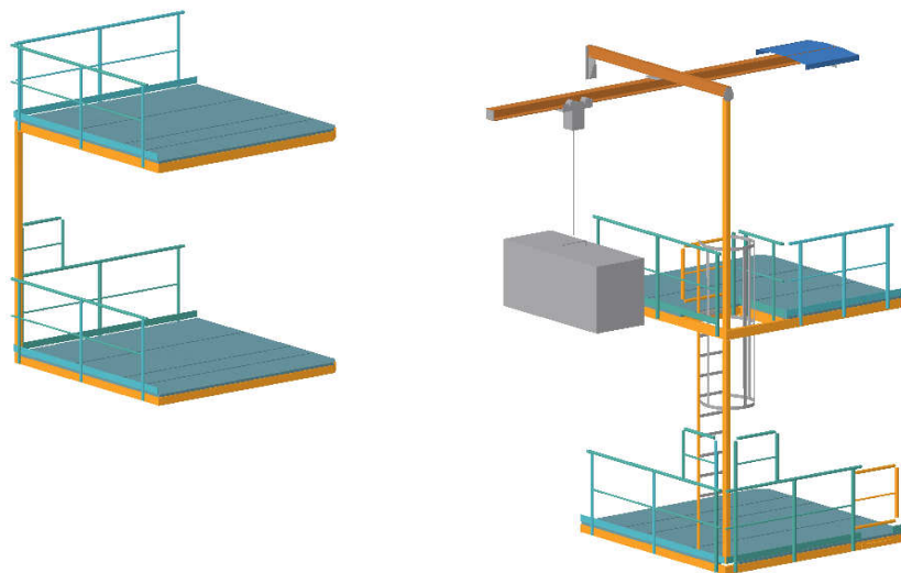
Рис. 3.38. Площадки обслуживания и грузовая лебедка КВОУ
