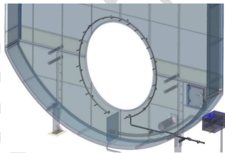
Рис. 3.37. Форсунки и трубопровод системы подачи ХОВ и моющего раствора в ГТУ
