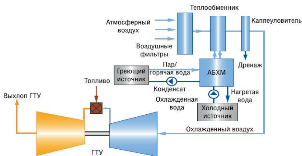
Рис.2.88. Принципиальная схема системы охлаждения циклового воздуха с АБХМ
