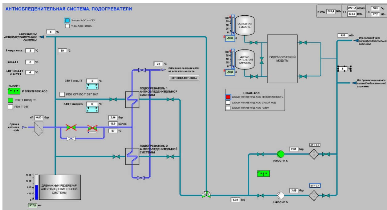
Рис. 3.23. Принципиальная схема АОС КВОУ ГТУ
