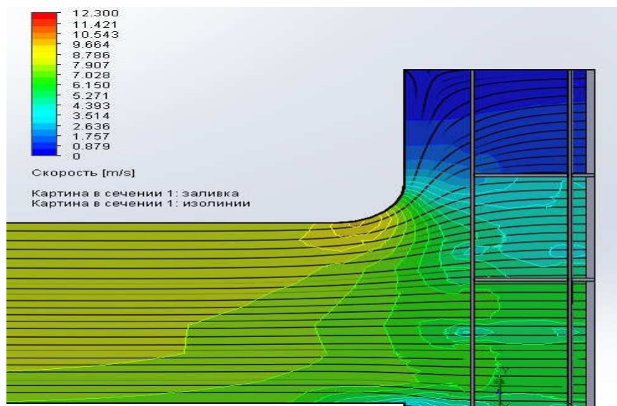
Рис. 5.16. Картина течения воздушного потока по высоте КВОУ ГТУ ТЭЦ в САО
