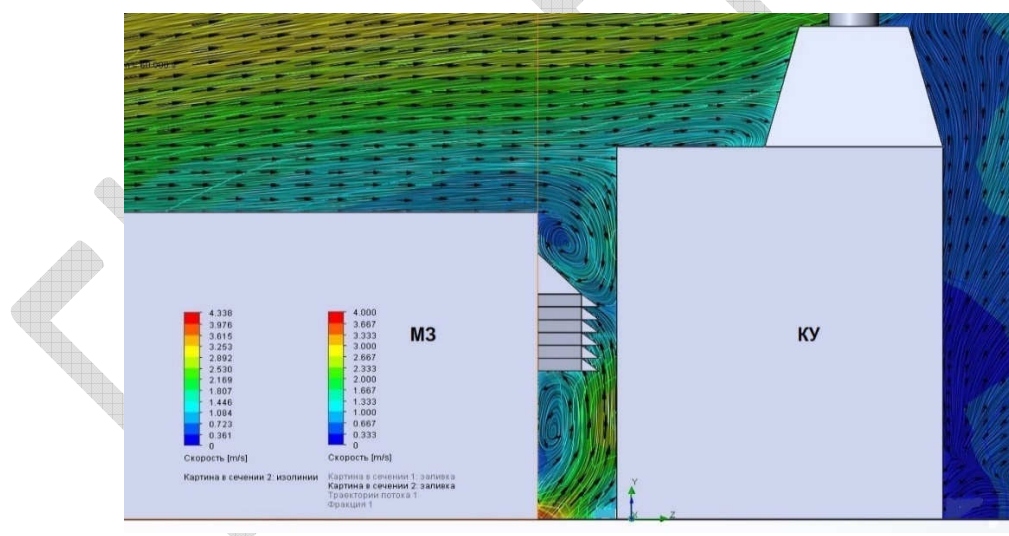
Рис. 5.7. Поле скоростей воздушного потока при западном направлении ветра
