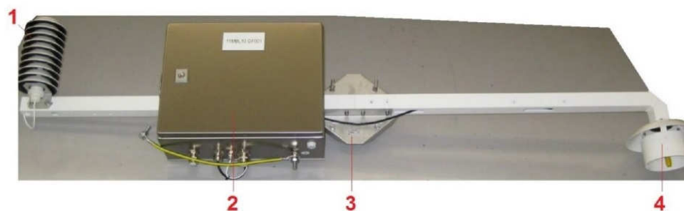
Рис. 3.43. Метеостанция КВОУ ГТУ: 1 – радиационный экран для дополнительного температурного зонда; 2 – передатчик; 3 – монтажная пластина для крепления; 4 – радиационный экран для зонда относительной влажности
