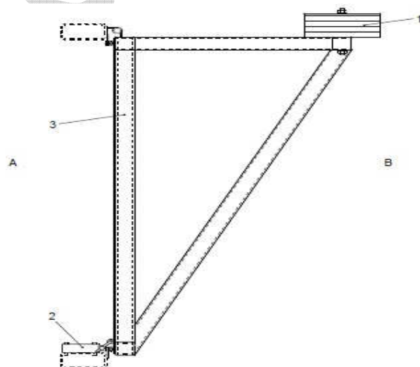
Рис. 3.39. Байпасный клапан: 1 – противовес; 2 – конечный выключатель; 3 – люк. А – зона окружающей среды; В – зона повышенного давления
