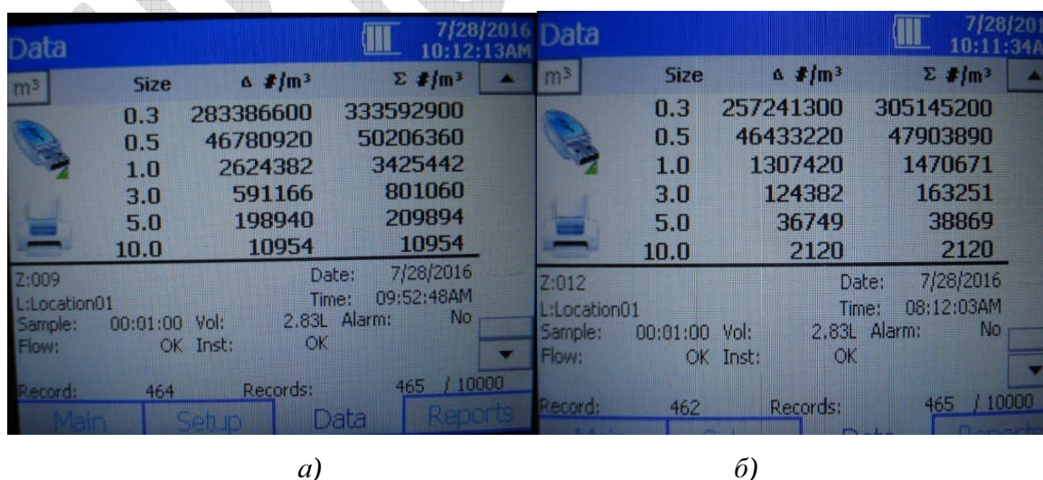
Рис. 4.13. Количество взвешенных частиц в кубометре атмосферного воздуха на всасе КВОУ ТЭЦ-1 в ЮАО (а), ТЭЦ в ЗАО (б)
