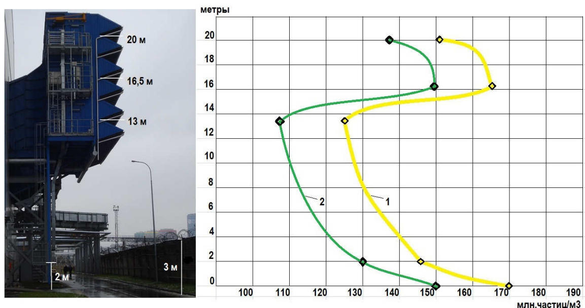
Рис. 4.2. Распределение количества взвешенных частиц в атмосферном воздухе по высоте КБОУ ТЭС в ЗАО: 1 – общее количество частиц; 2 – количество частиц размером 0,3–0,5 мкм
