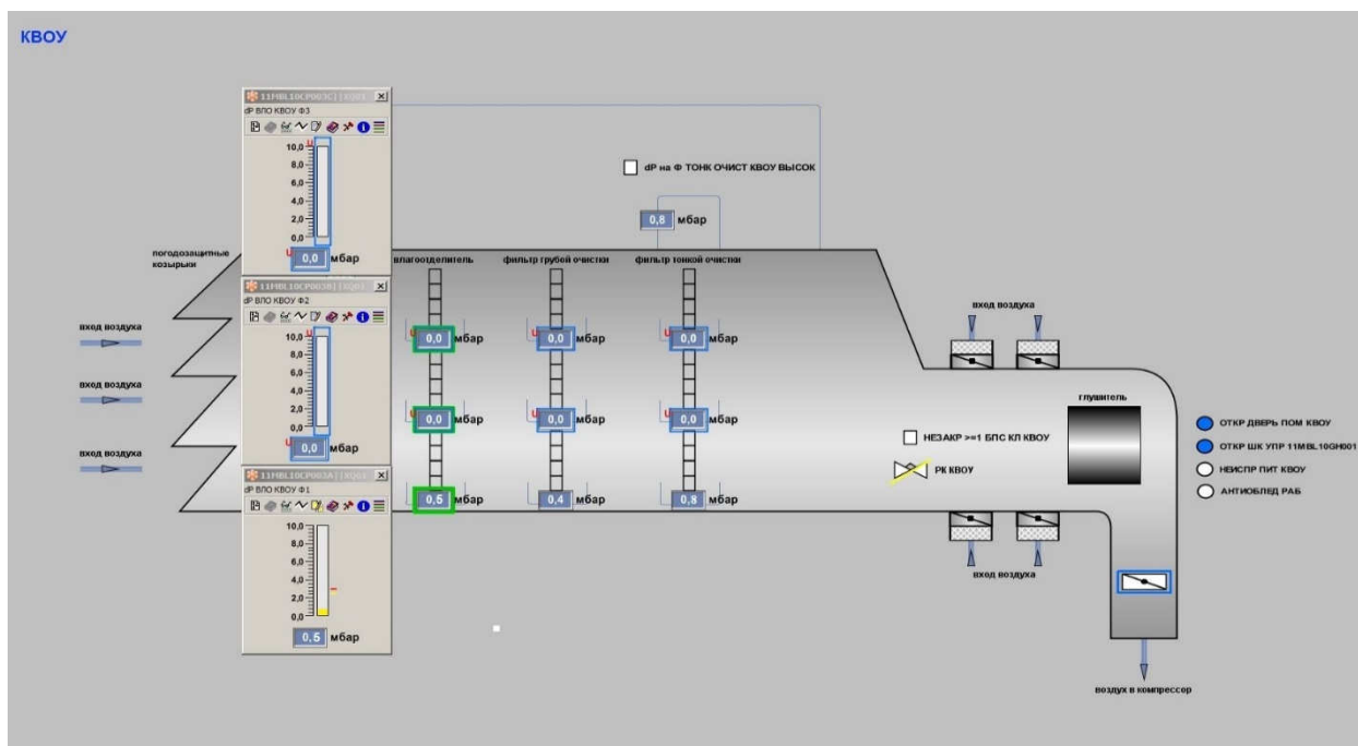
Рис. 4.35. Мнемокадр показаний датчиков давления на первом ярусе КВОУ ГТЭ-160
