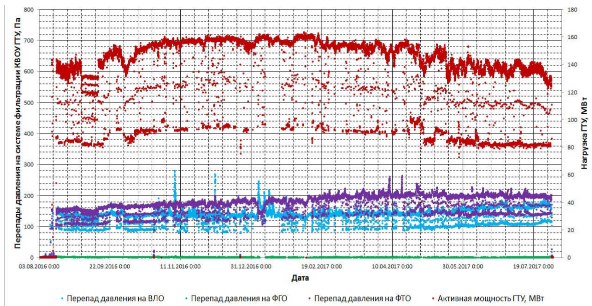
Рис. 4.24. Тренды перепадов давления на системе фильтрации КБОУ ГТУ-32 V94.2 ТЭЦ в МО в период с 04.08.2016 по 01.08.2017
