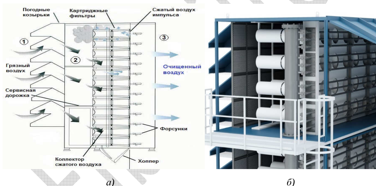
Рис. 3.3. КВОУ ГТУ с фильтрами импульсной очистки: а) принцип работы; б) 3D КВОУ (рис. из буклета компании Freudenberg Filtration Technologies)
