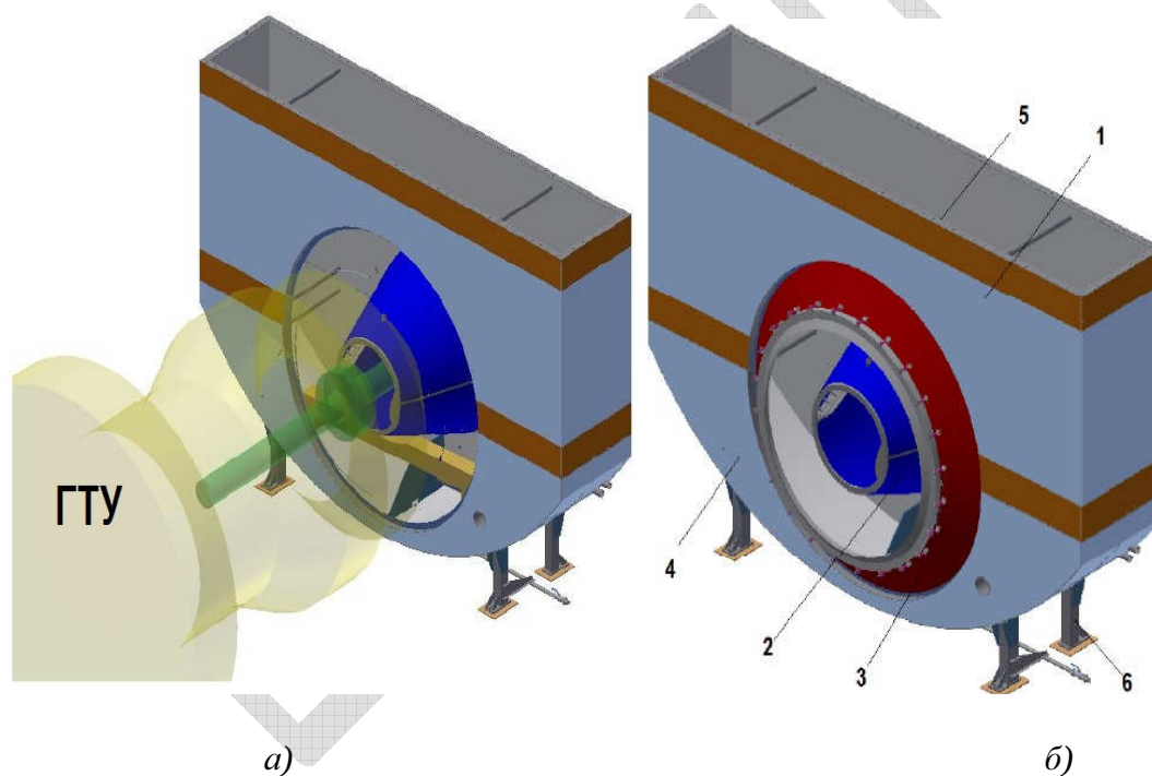
Рис. 3.35. Выходной воздуховод: а) соединение с ГТУ; б) конструкция: 1 – верхняя часть; 2 – внутренний конус; 3 – внешний конус; 4 – нижняя часть; 5 – раструб; 6 – опоры
