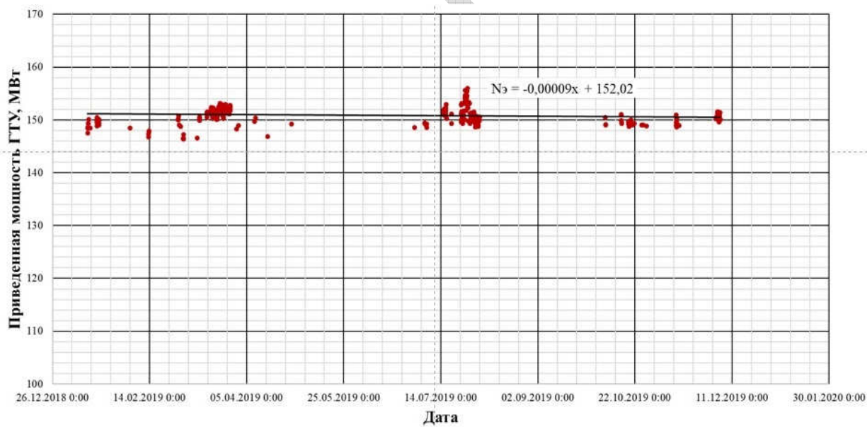
Рис. 4.33. Зависимость приведенной мощности ГТУ- 32 от наработки при ВНА 95%
