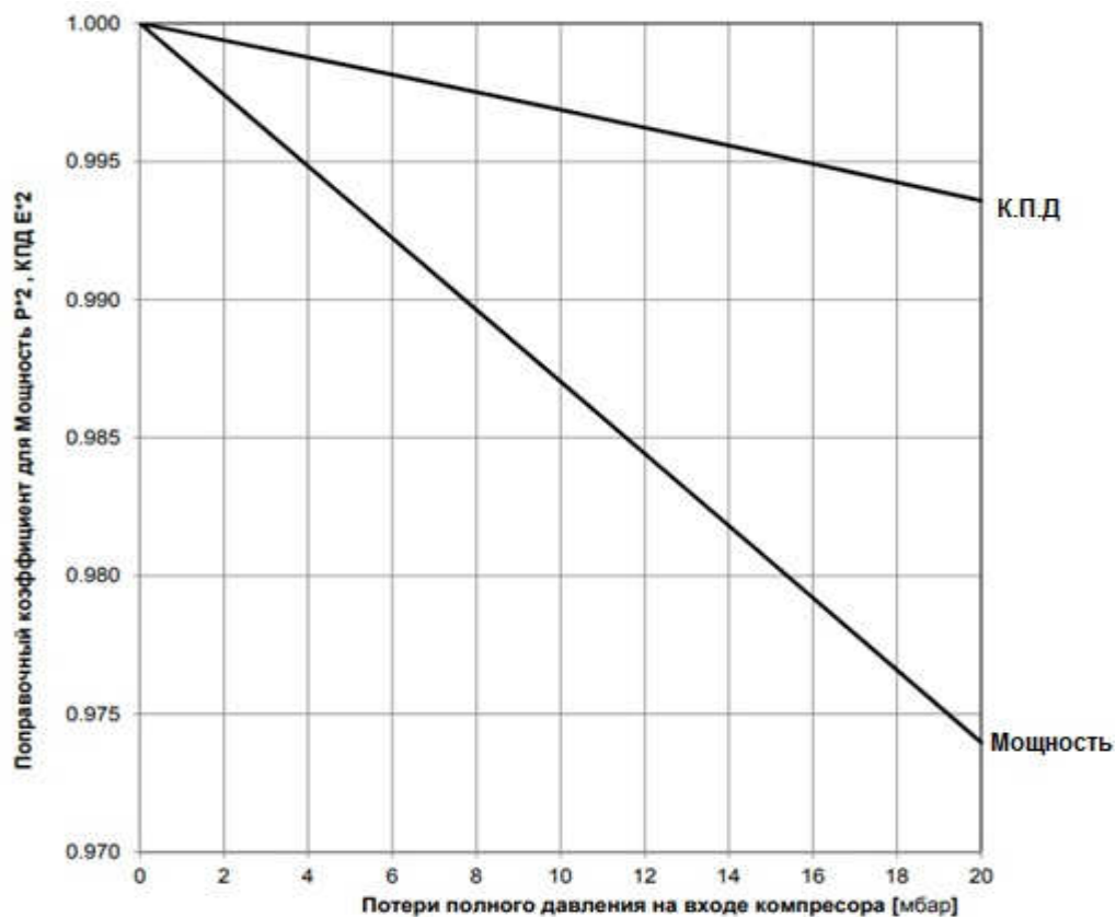
Рис. 2.78. Поправочные коэффициенты для мощности и КПД SGT5-4000F от потерь полного давления на входе в компрессор [19]
