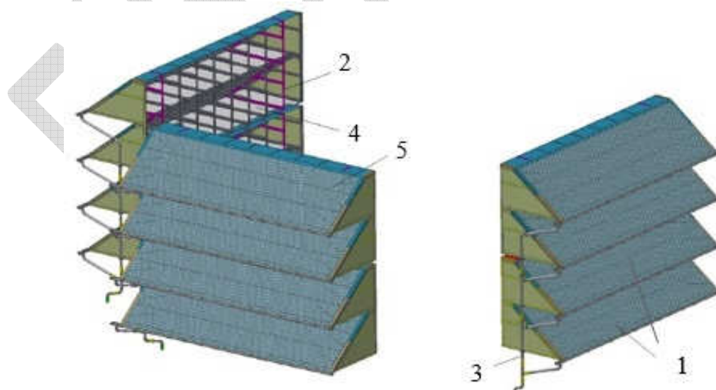
Рис. 3.22. Погодные козырьки: 1 – погодные козырьки; 2 – алюминиевые профильные балки; 3 – водосточный желоб; 4 – защитный экран от птиц; 5 – металлический обшивочный лист
