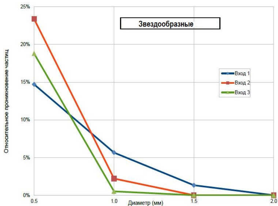
Рис. 2.17. Проникновение звездчатых снежинок на всас КВОУ по ярусам
