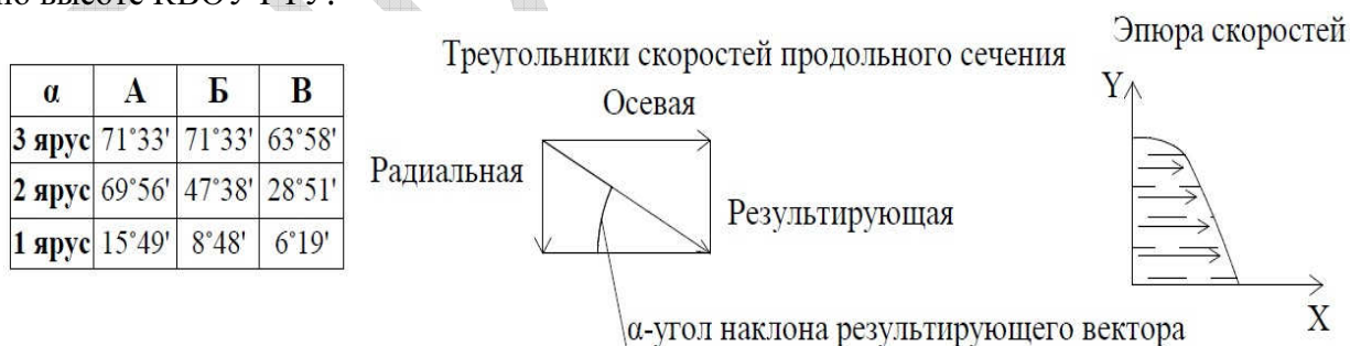
Рис. 5.33. Обозначения векторов скоростей и углов поворота потока, эпюра скоростей по высоте КВОУ ГТУ
