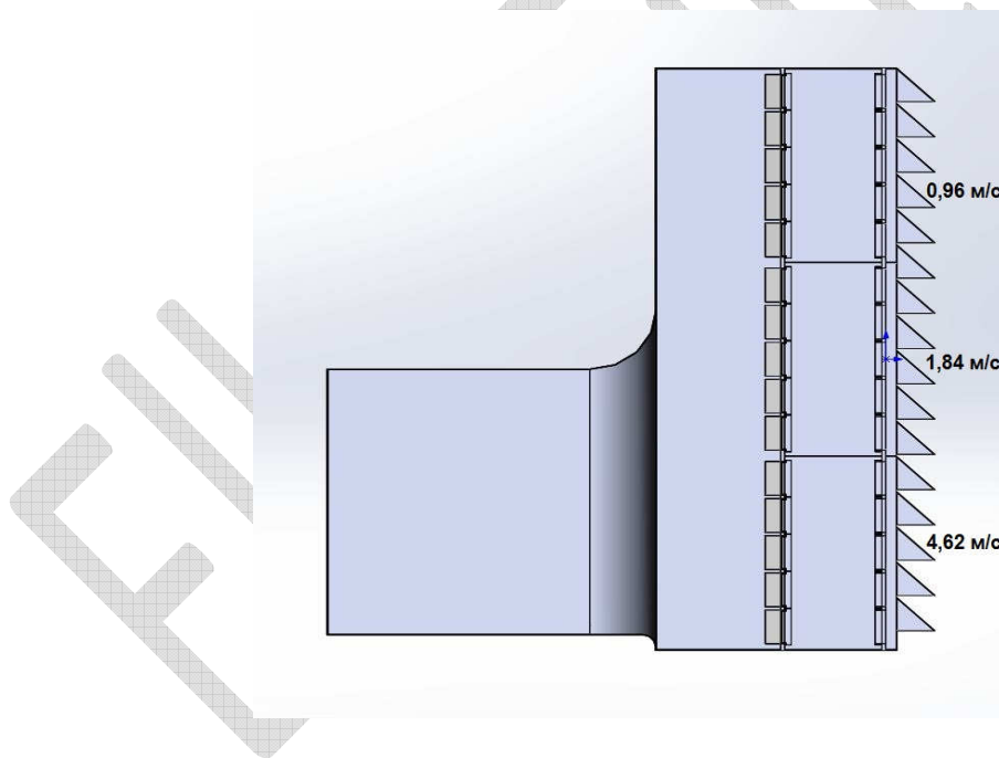
Рис. 5.15. Распределение скорости воздуха на всасе по высоте КВОУ ТЭЦ в CAO
