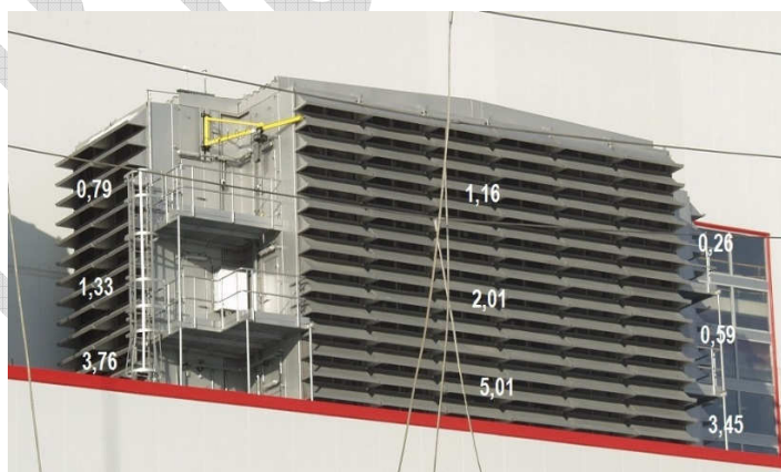
Рис. 5.21. Результаты замеров скорости на всасе КВОУ
