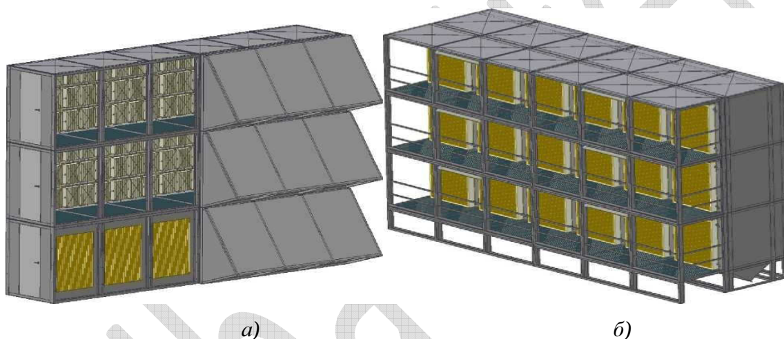
Рис. 3.18. КВОУ для ГТУ Siemens V64.3A, составленные из базовых модулей VARIPAC™: а) для статической; б) для импульсной очистки воздуха [5]
