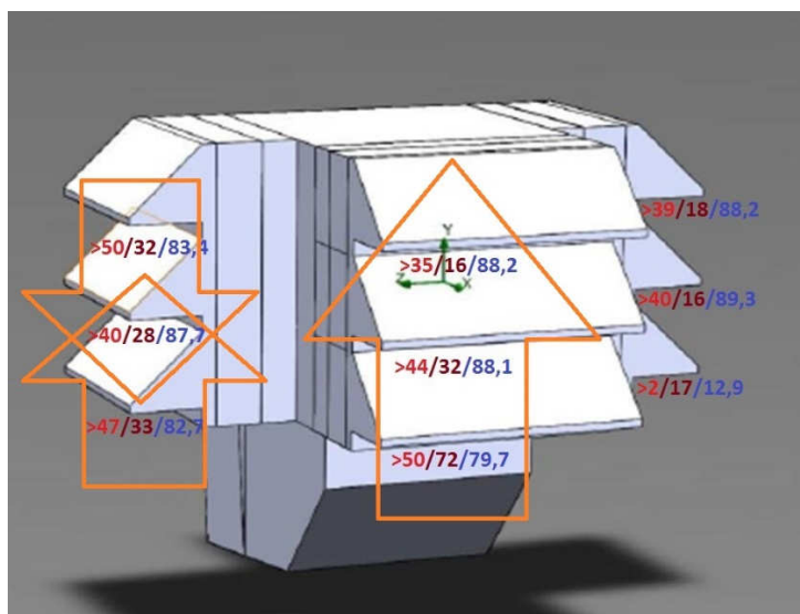
Рис. 5.25. Результаты замеров параметров атмосферного воздуха на КВОУ № 32: количество частиц \text{млн}/\text{м}^3 (красный цвет), концентрация частиц \text{мг}/\text{м}^3 (коричневый цвет); содержание мелкодисперсных частиц 0.3 \text{ мкм}/\text{м}^3 в процентах (синий цвет)
