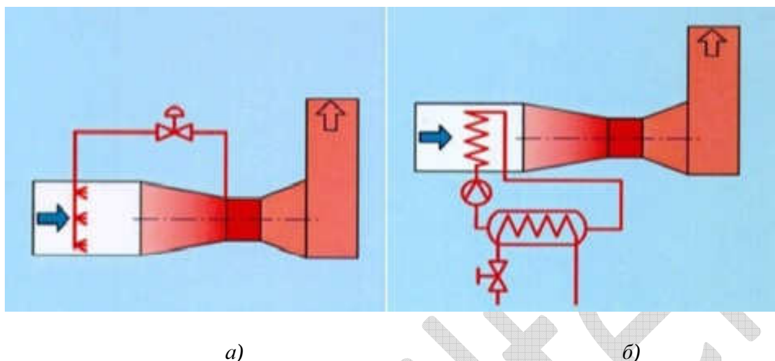
Рис. 2.66. Принципиальные схемы АОС: а) подача горячего воздуха из последних ступеней компрессора ГТУ; б) обогрев атмосферного воздуха в теплообменном аппарате
