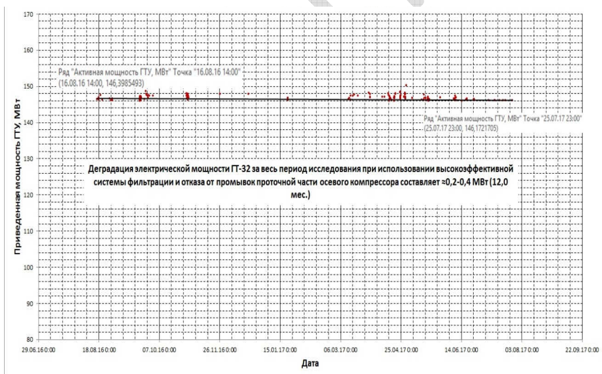
Рис. 4.25. График деградации приведенной мощности ГТУ-32 V94.2 ТЭЦ в МО вследствие загрязнения ОК при 87,0\% < BHA \leq 89,0\% ; АОС выкл. ( t_{HK} - t_{H6} \leq 1,5 °C)
