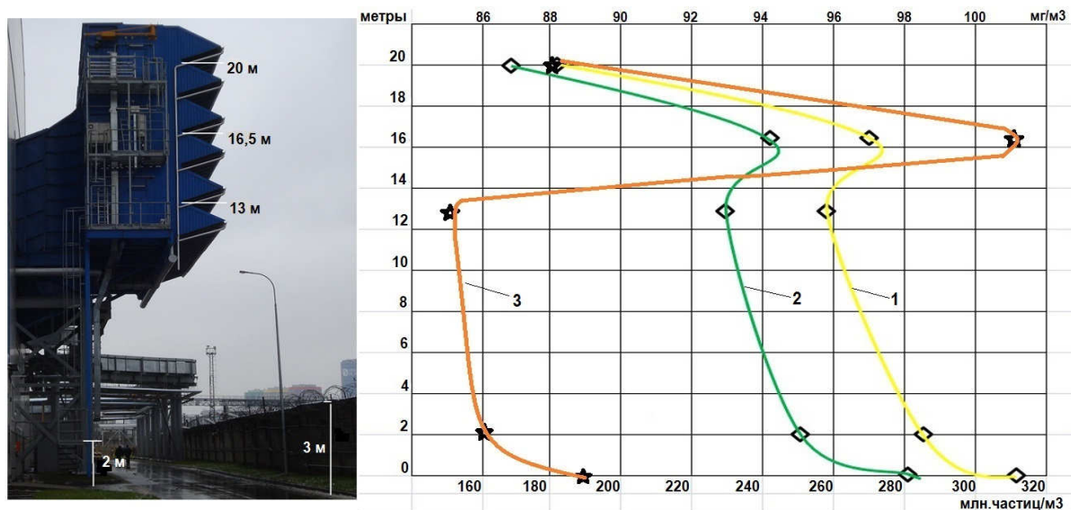
Рис. 4.5. Распределение количества и концентрации взвешенных частиц в кубометре атмосферного воздуха по высоте КВОУ (29.03.2016): 1 – суммарное количество взвешенных частиц; 2 – количество мелкодисперсных частиц (0,3 мкм); 3 – суммарная концентрация взвешенных частиц
