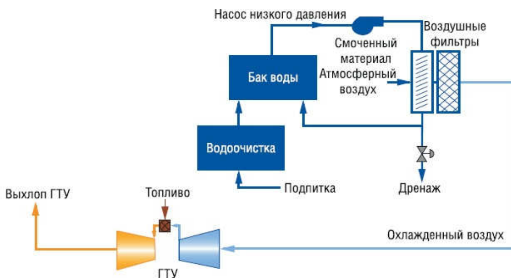
Рис. 2.84. Схема работы ОУ ИТ
