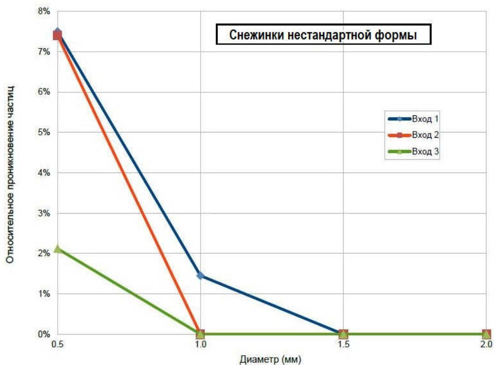
Рис. 2.18. Проникновение нестандартной формы на всас КВОУ по ярусам
