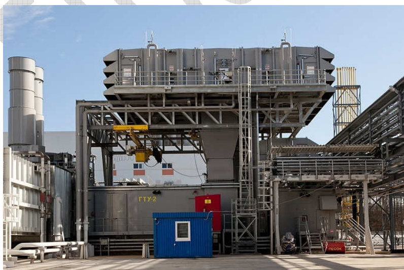
Рис. 3.6. КБОУ ГТУ LMS 100 PB Джубгинской ТЭС ( https://clck.ru/33anno )
