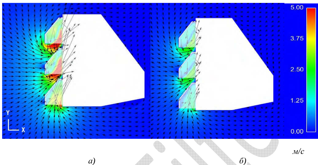
Рис. 2.11. Величина и векторы скорости по оси X при расходе: а) 130 кг/с; б) 65 кг/с
