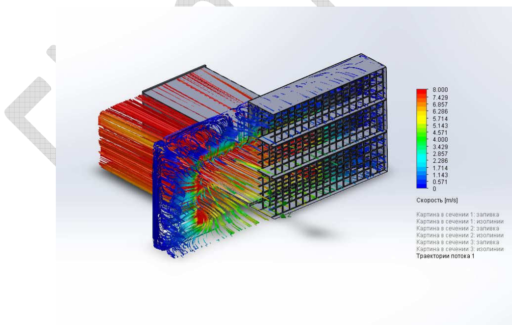
Рис. 5.18. Поле скоростей воздушного потока в КВОУ и воздуховоде ГТУ
