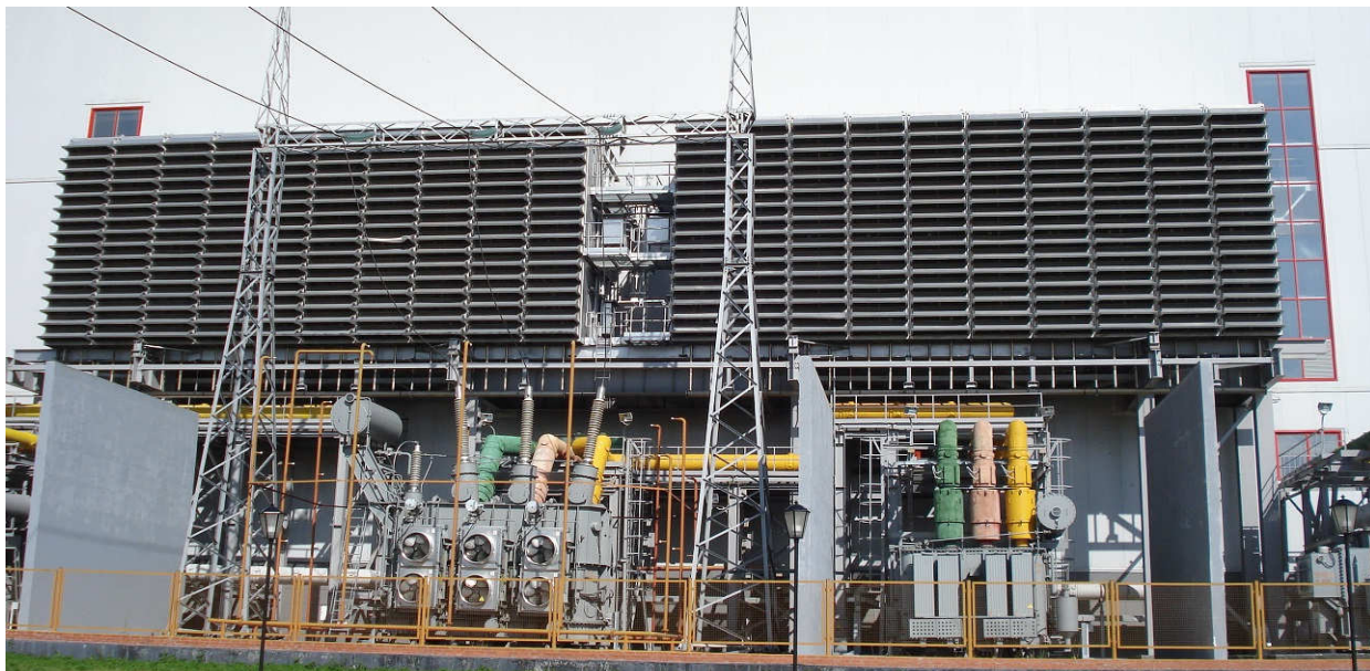
Рис. 5.36. КВОУ ГТУ и силовые трансформаторы энергоблока ПГУ
