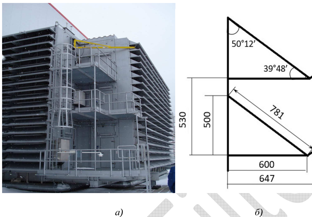
Рис. 2.23. КВОУ Camfil Farr: а) погодные козырьки; б) размеры погодных козырьков
