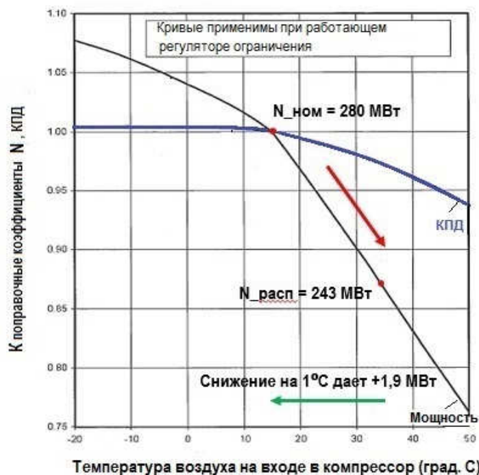
Рис. 2.82. Зависимость выходной мощности и КПД ГТУ Siemens SGT5-4000F от температуры наружного воздуха
