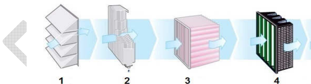
Рис. 3.10. Система фильтрации циклового воздуха ГТУ: 1 – погодные козырьки, 2 – жалюзийный каплеуловитель, 3 – карманный ФГО/ФСО, 4 – кассетный ФТО (рис. из буклета компании Camfil Svenska)
