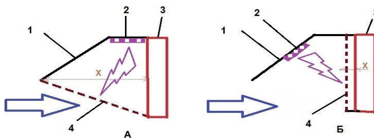
Рис. А- КВОУ с наклонной защитной сеткой от птиц Рис. Б- КВОУ с вертикальной защитной сеткой от птиц
