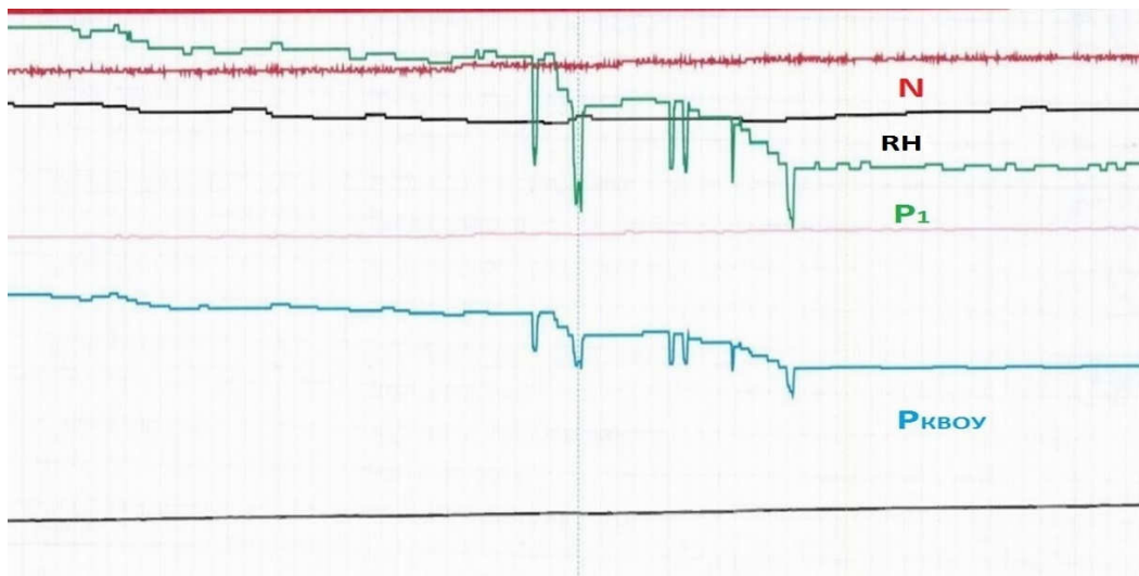
Рис. 2.53. Тренды изменения давления на фильтрах-коагуляторах и КВОУ ГТУ [15]
