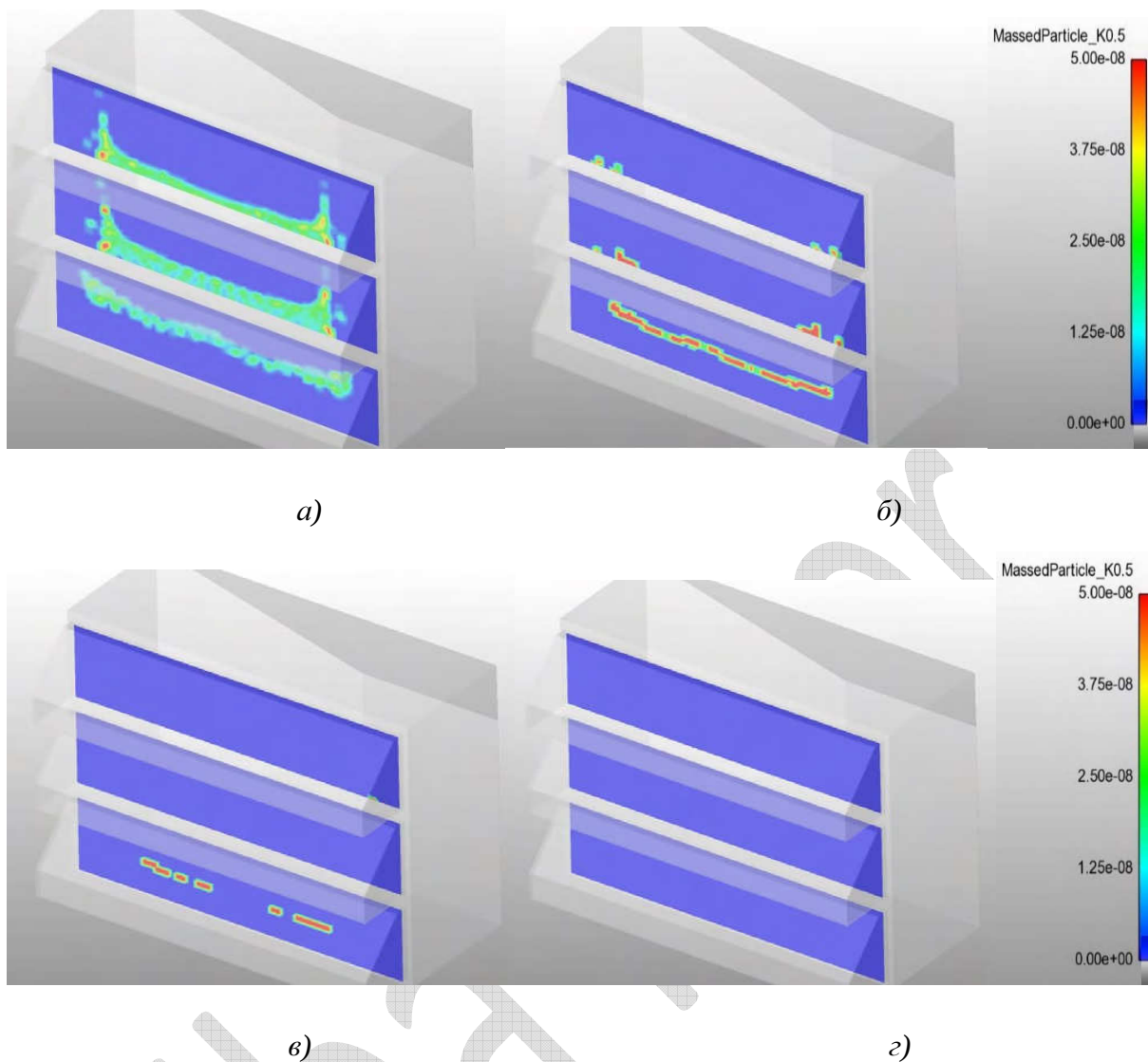
Рис. 2.14. Распределение масс снежинок в виде звезд по их размерам в погодных козырьках по высоте КВОУ: а) 0,5 мм; б) 1,0 мм; в) 1,5 мм; г) 2,0 мм
