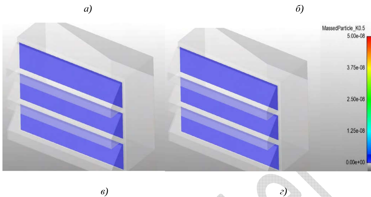
Рис. 2.15. Распределение масс снежинок нерегулярных форм по их размерам в погодных козырьках по высоте КВОУ: а) 0,5 мм; б) 1,0 мм; в) 1,5 мм; г) 2,0 мм
