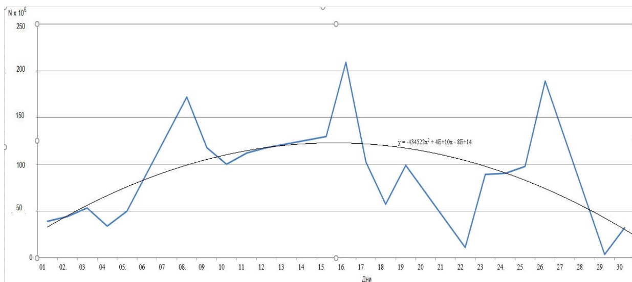
Рис. 4.18. Максимальное количество частиц в кубическом метре атмосферного воздуха на всасе КВОУ ГТУ ТЭЦ-1 в ЮАО в июне 2020 года
