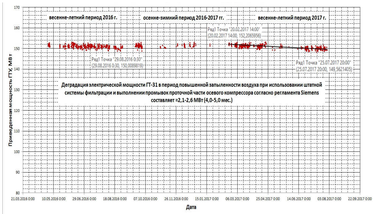
Рис. 4.28. График деградации приведенной мощности ГТУ-31 V94.2 ТЭЦ в МО вследствие загрязнения ОК при 87,0\% < \text{ВНА} \leq 89,0\% ; АОС выкл. ( t_{\text{нк}} - t_{\text{не}} \leq 1,5^\circ\text{C} )
