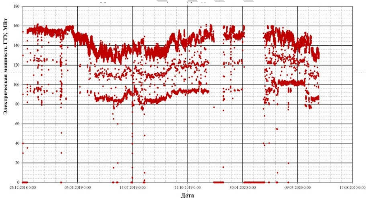
Рис. 4.31. Тренды нагрузки на ГТУ-32 ТЭЦ в МО
