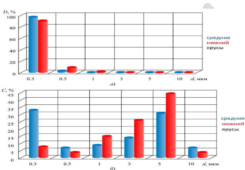
Рис. 4.8. Дисперсность D (а) и распределение концентрации C (б) взвешенных частиц в атмосферном воздухе на нижнем и средних ярусах КВОУ ГТУ ТЭЦ-2 в ЮАО
