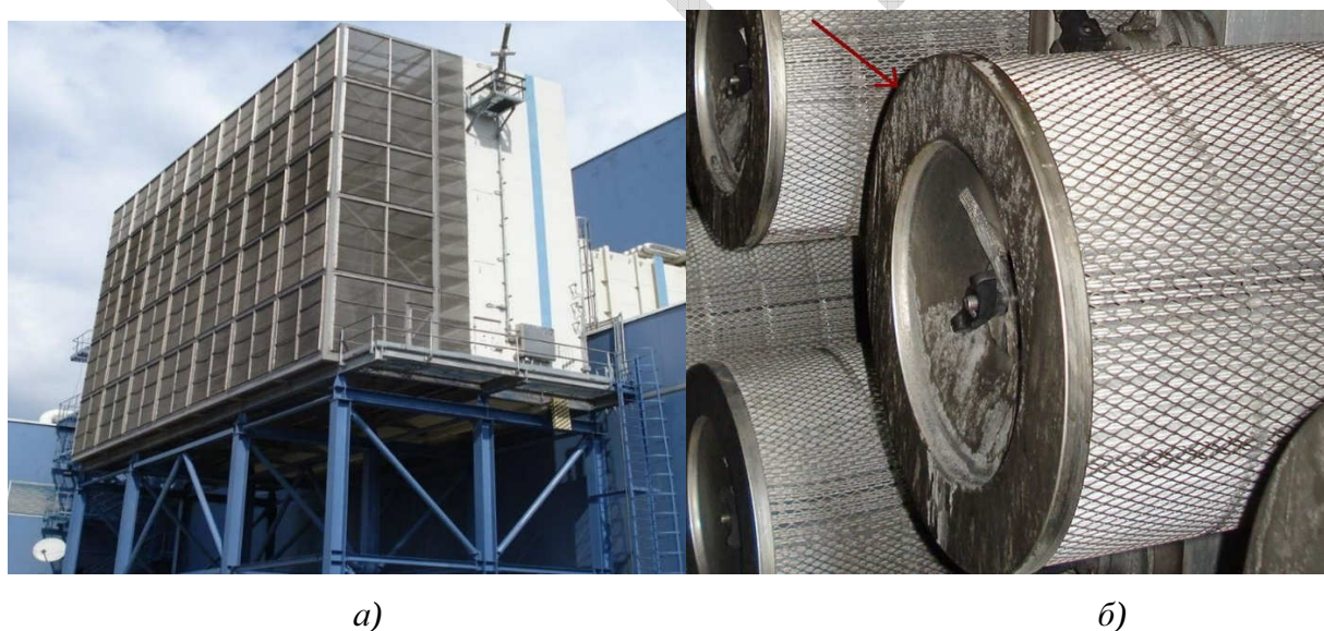
Рис. 3.7. КВОУ и фильтры ГТУ PG935FA GE: а) КВОУ Шатурской ГРЭС; б) импульсные фильтры КВОУ Сургутской ГРЭС-2
