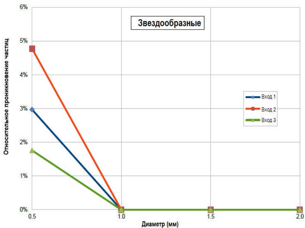
Рис. 2.20. Проникновение звездообразных снежинок на всас КВОУ по ярусам
