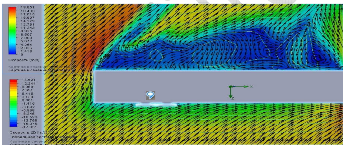
Рис. 5.12. Картина натекания потока воздуха южным направлением ветра на КБОУ при расчетной скорости ветра 12 м/с по программе Solid Works Flow Simulation
