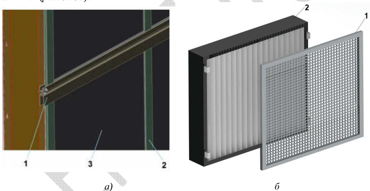
Рис. 3.25. Способы крепления противомоскитных сеток: а) 1 – алюминиевый профиль, 2 – пластиковый Н-образный профиль, 3 – противомоскитная сетка; б) 1 – противомоскитная сетка; 2 – фильтр
