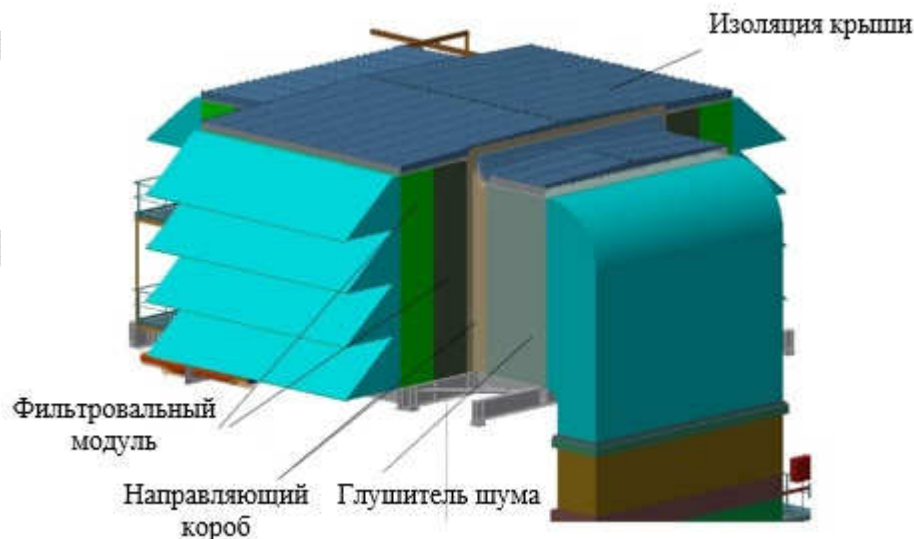
Рис. 3.21. Общий вид ВЗТ с коротким горизонтальным воздуховодом
