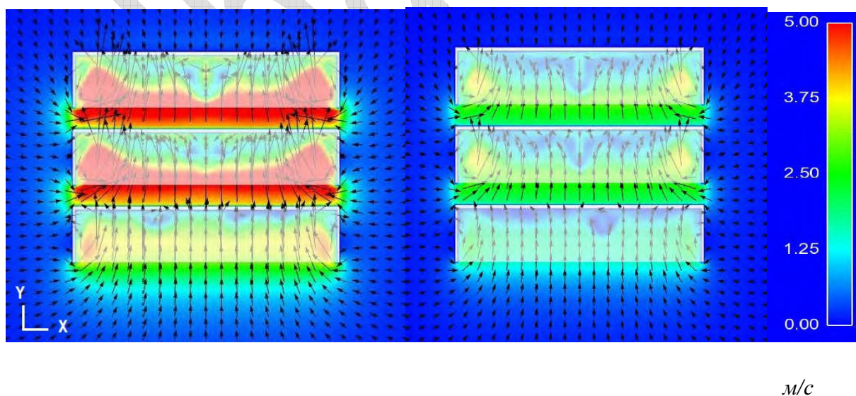
Рис. 2.12. Величина и вектора скорости по оси Y при расходе: а) 130 кг/с; б) 65 кг/с
