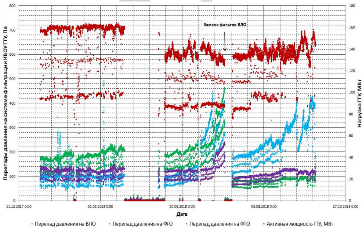
Рис. 4.27. Тренды перепадов давления на системе фильтрации КВОУ ГТУ-31 V94.2 ТЭЦ в МО с 01.01.2018 по 28.09.2018
