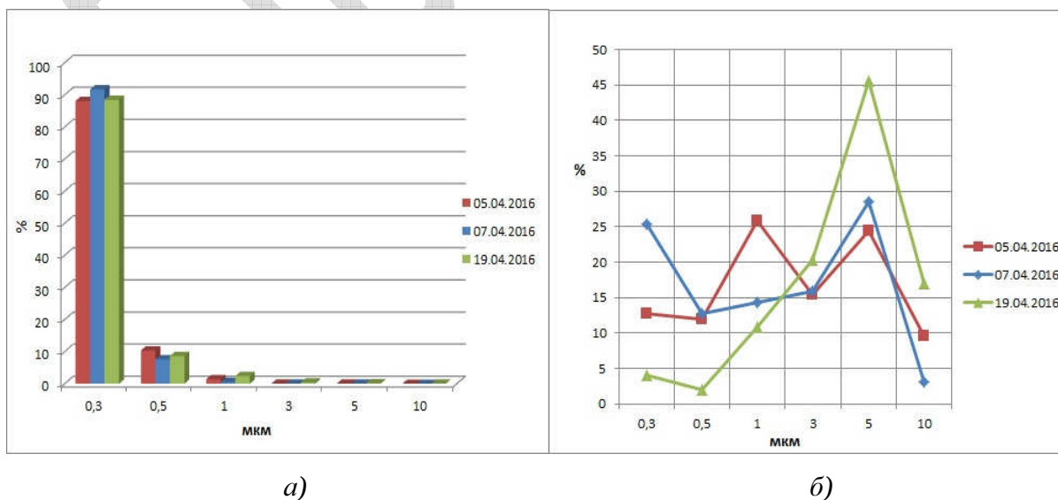
Рис. 5.24. Процентное распределение частиц в кубометре атмосферного воздуха по дисперсности: а) количество; б) концентрация
