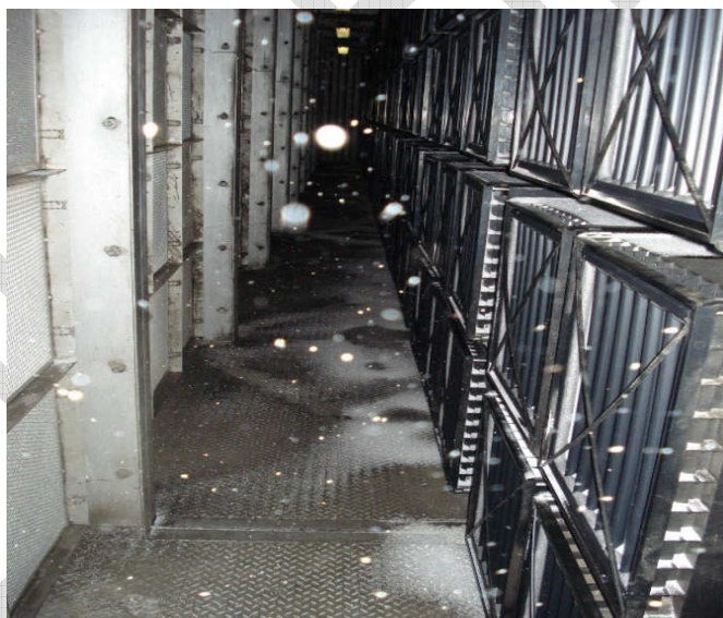
Рис. 2.24. Проникновение снежинок в КВОУ ГТУ
