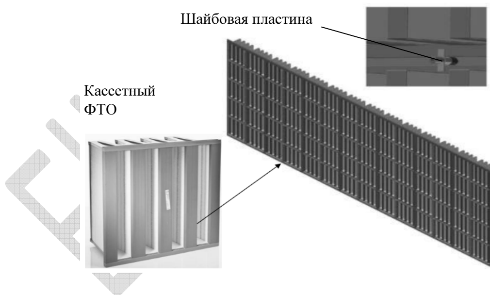
Рис. 3.28. Фильтры тонкой очистки
