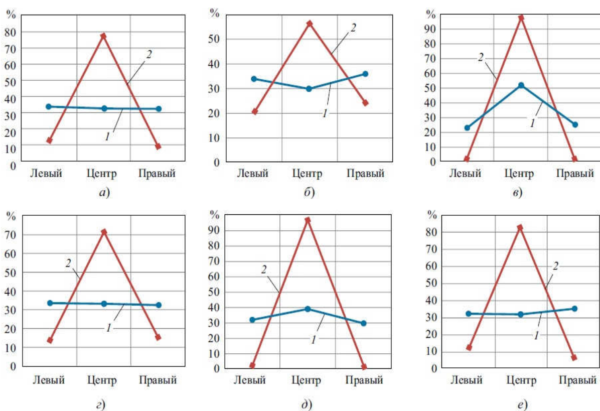
Рис. 5.3. Процентное распределение количества (1) и концентрации (2) взвешенных частиц в кубометре атмосферного воздуха по всасам КВОУ: а) 02.11.2015; б) 04.05.2016; в) 13.05.2016; г) 03.06.2016; д) 09.01.2017; е) 11.05.2017
