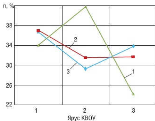
Рис. 2.28. Распределение взвешенных частиц в атмосферном воздухе по ярусам КВОУ: 1 – 25.05.2020; 2 – 29.05.2020; 3 – 28.05.2020
