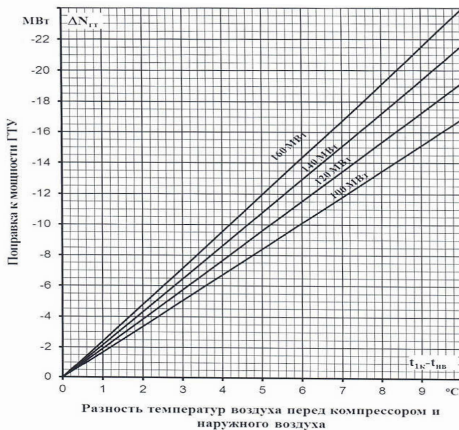
Рис. 2.71. Поправка мощности ГТЭ-160 на включение АОС [18]
