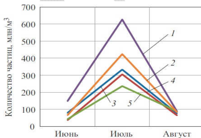
Рис. 4.15. Количество взвешенных частиц на всасах КВОУ ТЭЦ: 1 – ТЭЦ в ЮЗАО; 2 – ТЭЦ в МО; 3 – ТЭЦ-1 в ЮАО; 4 – ТЭЦ в ЗАО; 5 – ТЭЦ в СЗАО
