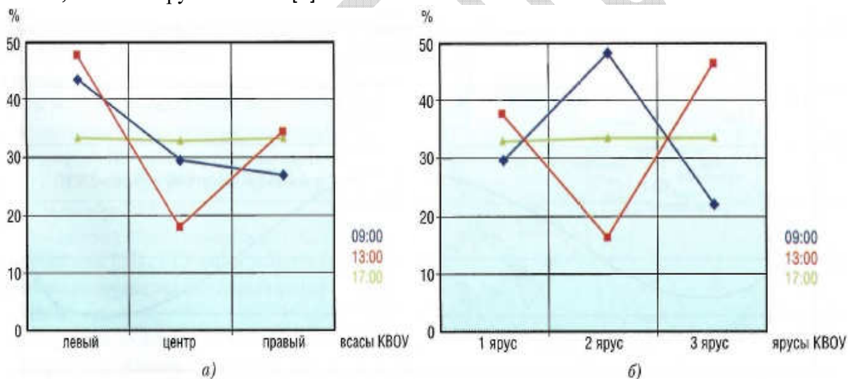
Рис. 4.17. Процентное распределение максимального количества частиц в кубометре атмосферного воздуха на ТЭЦ СЗАО: а) по всасам КВОУ; б) по ярусам КВОУ
