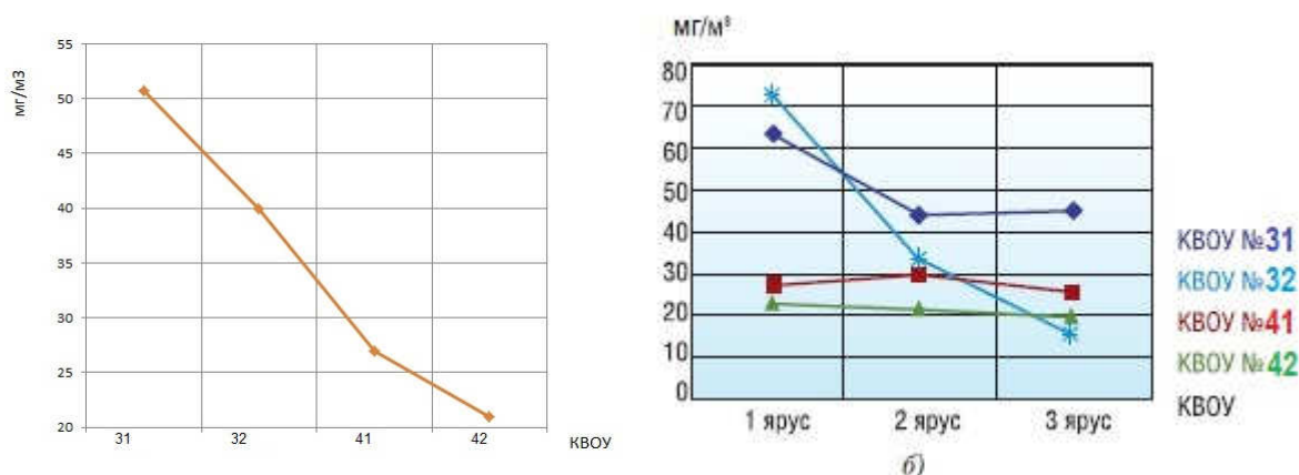
Рис. 5.28. Распределение концентрации частиц в кубометре атмосферного воздуха: а) по всасам; б) по ярусам КБОУ
