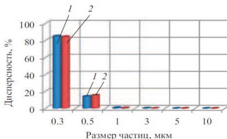
Рис. 4.14. Распределение дисперсности взвешенных частиц атмосферного воздуха на всасе КВОУ ТЭЦ-1 в ЮАО (1) и ТЭЦ в ЗАО (2) 28 июля 2016 года
