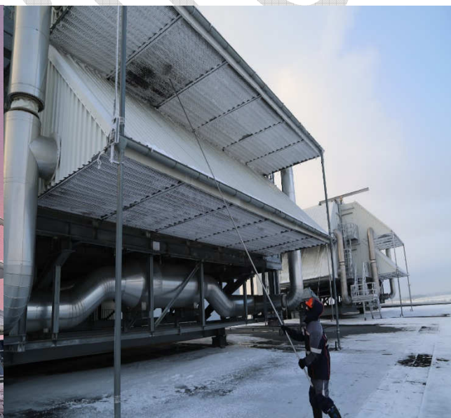
Рис. 2.52. Очистка защитных сеток от птиц на КВОУ ГТЭ-160 ООО «Хуадянь-Тенинская ТЭЦ»
