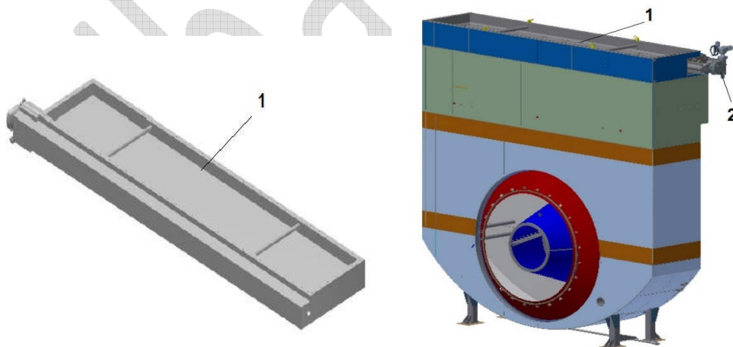
Рис. 3.34. Запорная заслонка: 1 – внешний вид и место установки; 2 – электропривод
