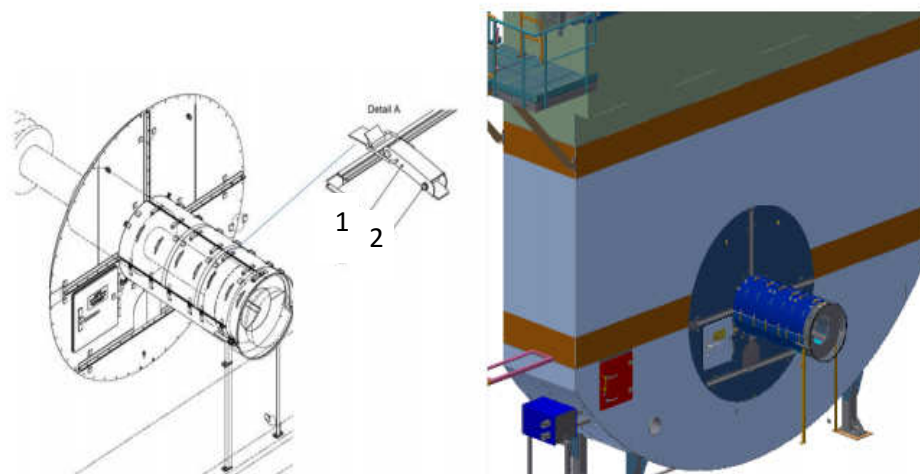
Рис. 3.36. Защита вала генератора: 1 – зажим; 2 – предохранительные винты и болты
