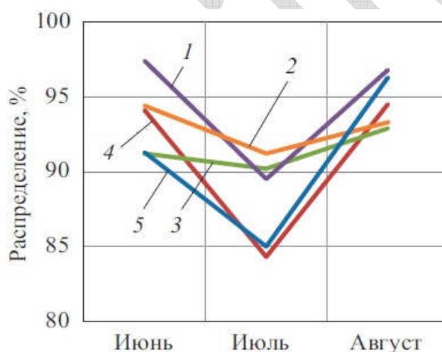
Рис. 4.16. Сравнение ТЭЦ с ГТУ по распределению мелкодисперсных частиц (0,3–0,5 мкм) в кубометре атмосферного воздуха на всах КВОУ: 1 – ТЭЦ в ЮЗАО; 2 – ТЭЦ в МО; 3 – ТЭЦ в СЗАО; 4 – ТЭЦ ЗАО; 5 – ТЭЦ-1 в ЮАО
