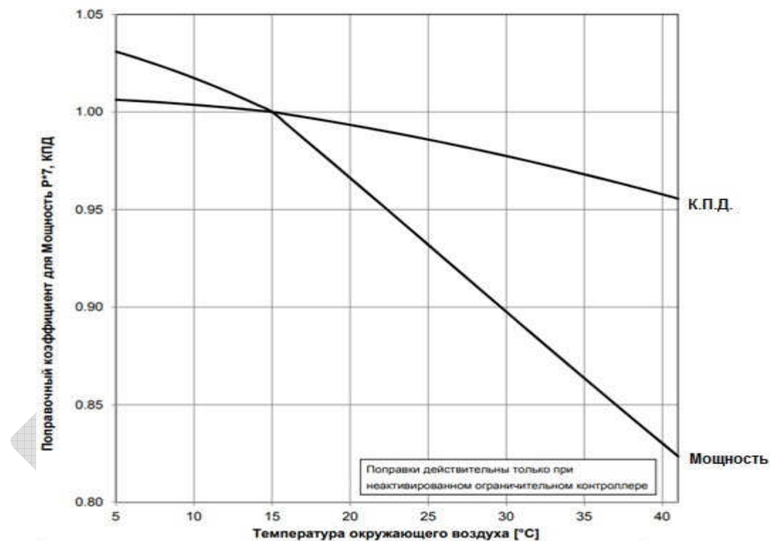
Рис. 2.77. Поправочные коэффициенты для мощности и КПД SGT5-4000F от температуры воздуха [19]
