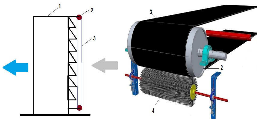
Рис. 2.38. Техническое решение по установке штатных противомоскитных сеток [9]: 1 – КВОУ; 2 – барабаны; 3 – двухсторонняя противомоскитная сетка; 4 – щетка
