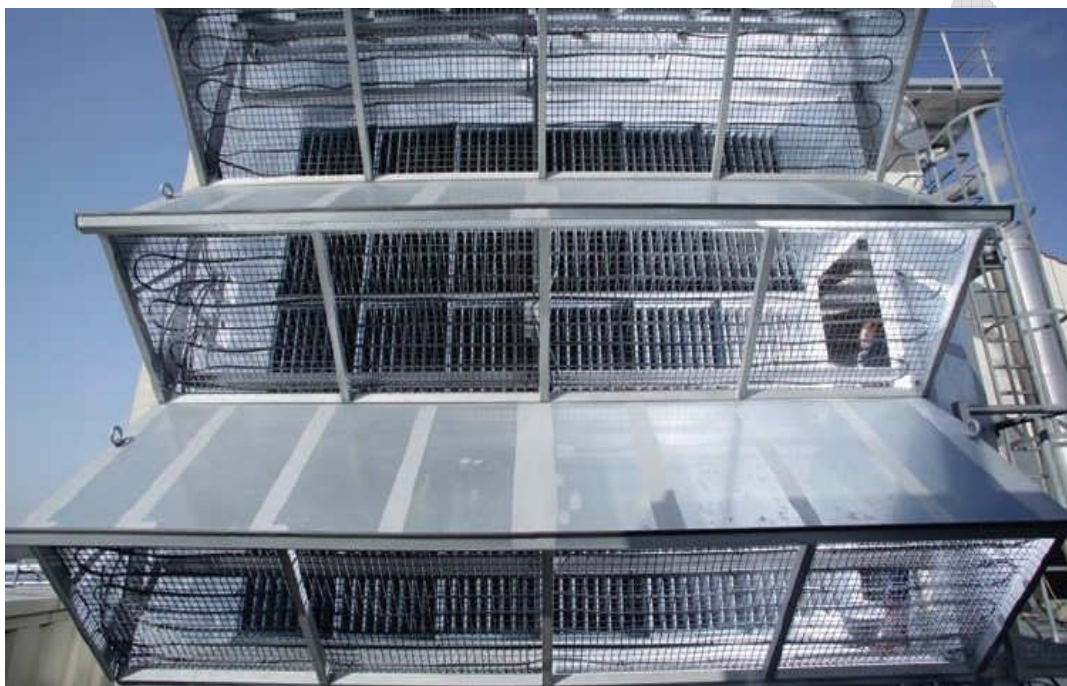
Рис. 2.58. АОС КВОУ ГТУ SolarTaurus70 с саморегулирующимся греющим электрическим кабелем [15]
