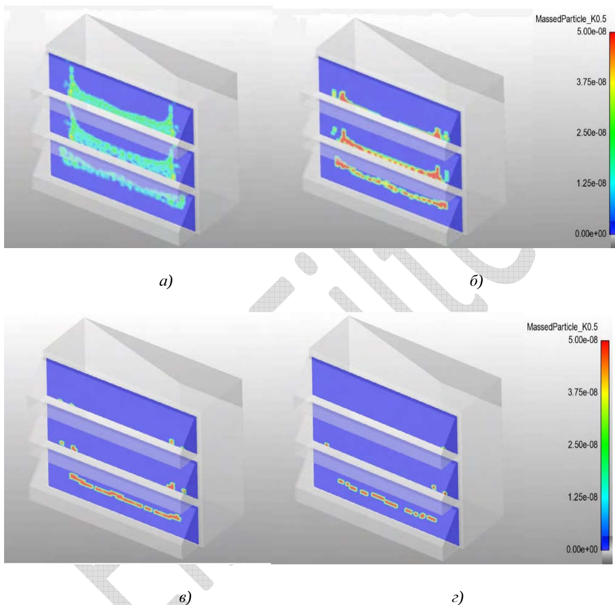
Рис. 2.13. Распределение масс снежинок в виде пластин по их размерам в погодных козырьках по высоте КВОУ: а) 0,5 мм; б) 1,0 мм; в) 1,5 мм; г) 2,0 мм
