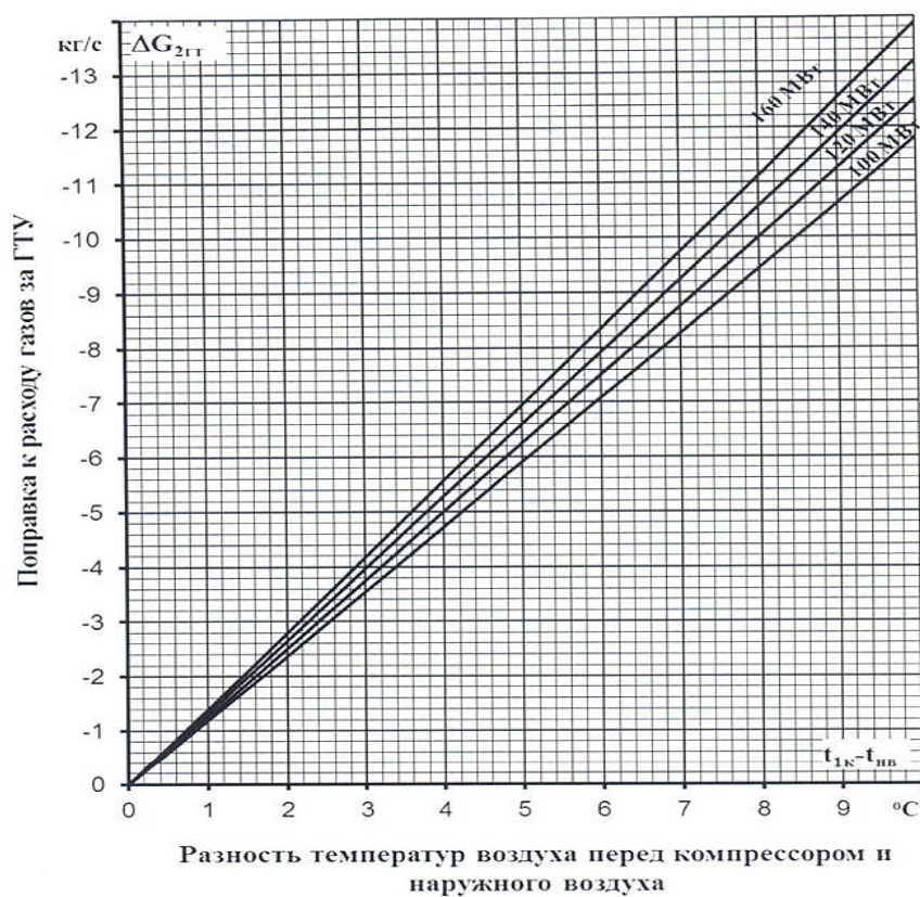
Рис. 2.72. Поправка расхода газов ГТЭ-160 на включение АОС [18]
